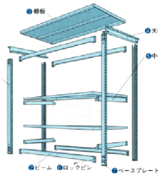
●1台当り部材(5段仕様)
